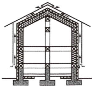
付加断熱 (外+充填断熱)
